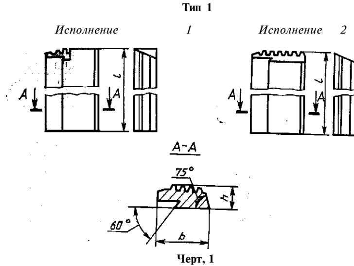
Гребенки для метрической резьбы мм
